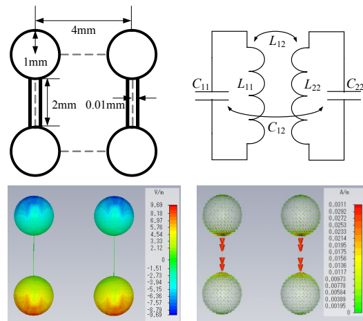
図 2 : 簡単な構造の等価回路と電荷・電流分
